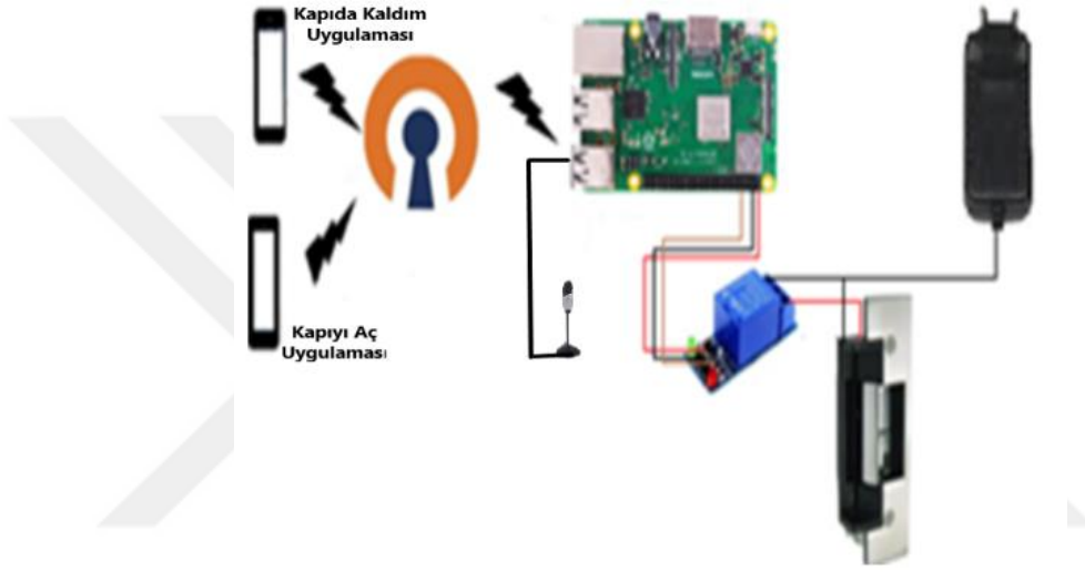
Şekil 5.1. Sistemin genel yapısı
